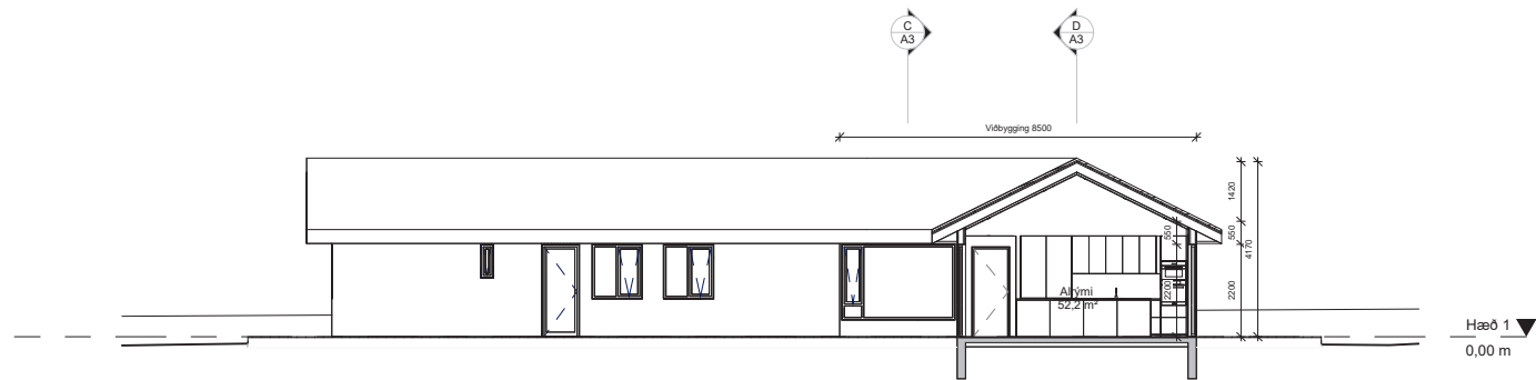
Snið A 1:100
